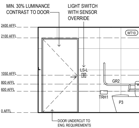
RACF - ACCESSIBLE ENSUITE ELEVATION 1 Scale 1 : 50
