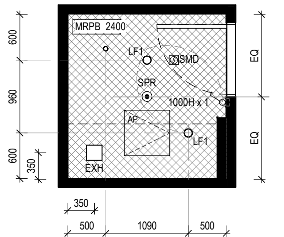
2 RCP-STANDARD ENSUITE Scale 1 : 50
