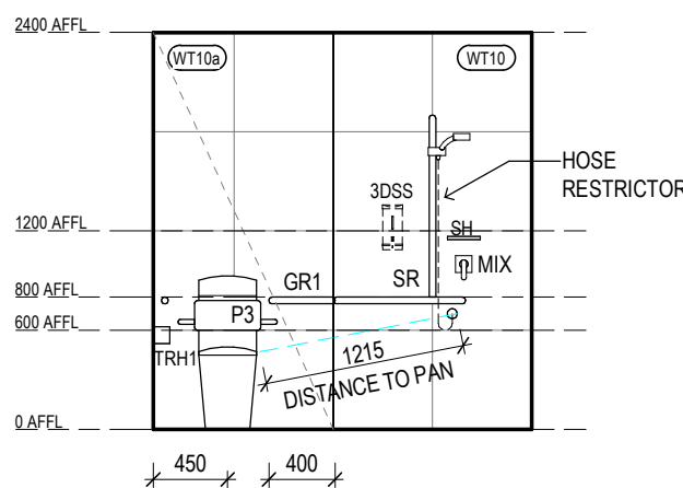
RACF - ACCESSIBLE ENSUITE ELEVATION 4 Scale 1 : 50
