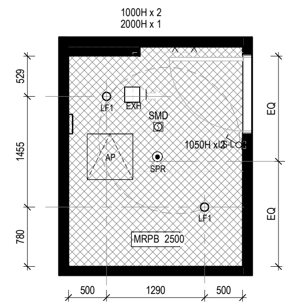
4 RCP - ACCESSIBLE BEDROOM Scale 1 : 50
